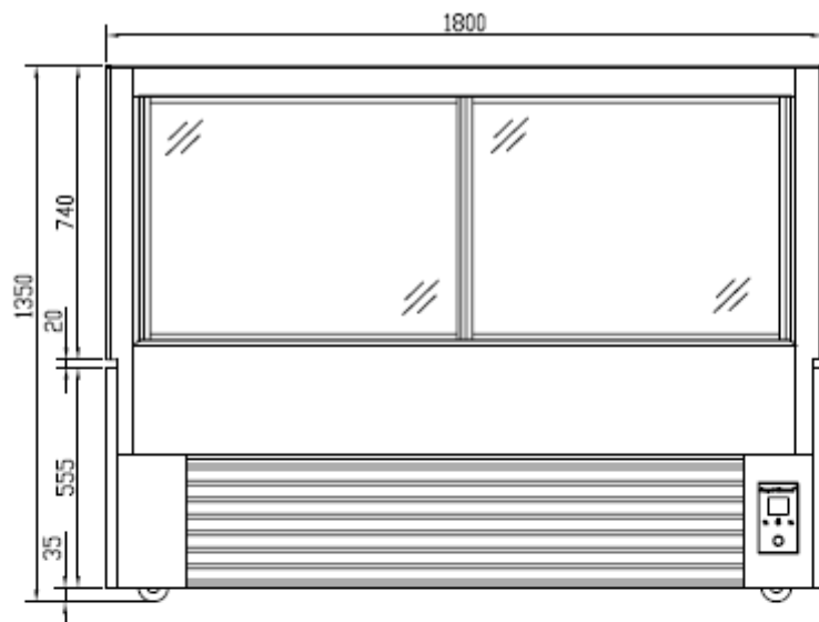
BACK 后视图
