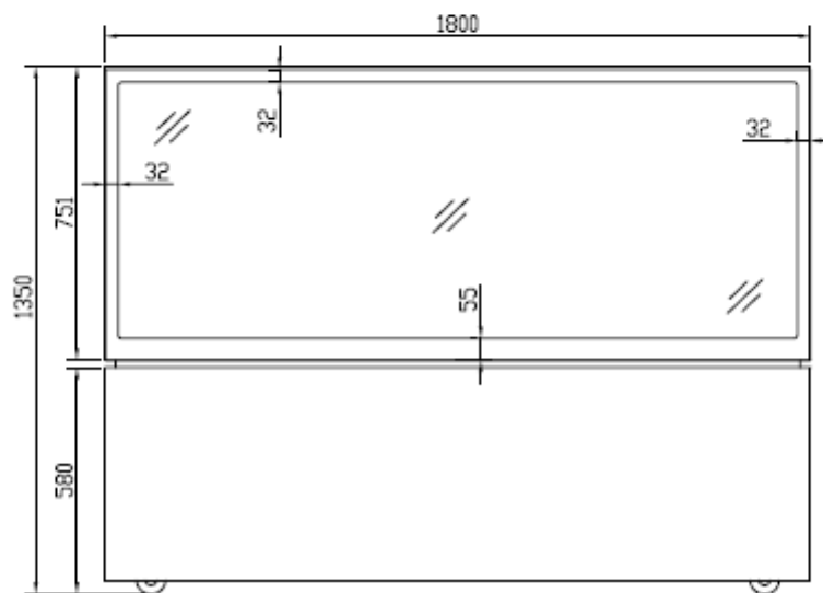
ELEVATION 前视图
