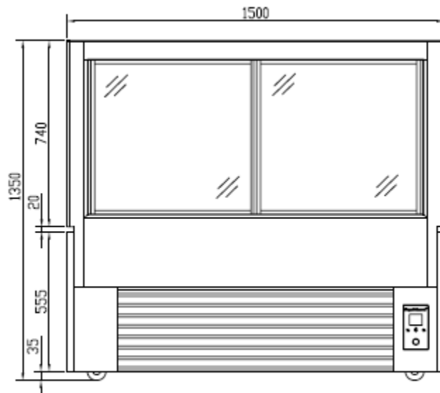
BACK 后视图
