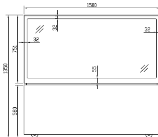
ELEVATION 前视图
