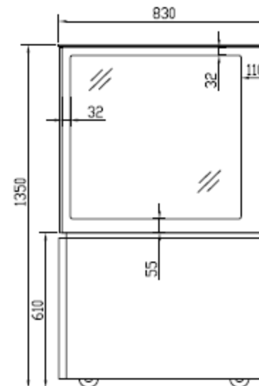
SIDE VIEW 左视图
