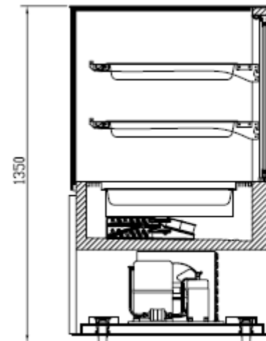
SECTION VIEW 左半剖视图
