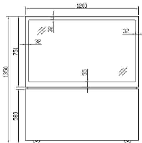
ELEVATION 前视图
