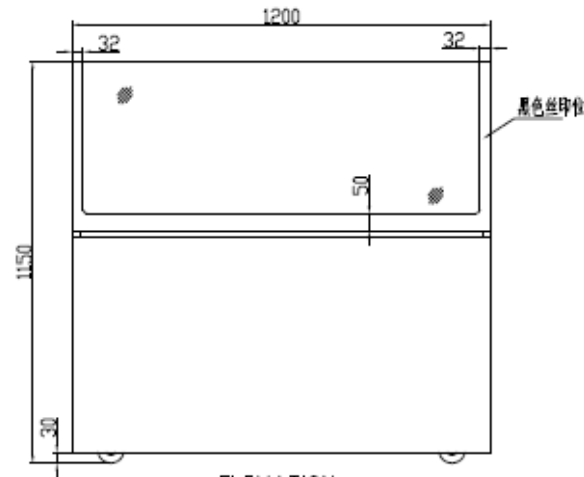
ELEVATION 前视图
