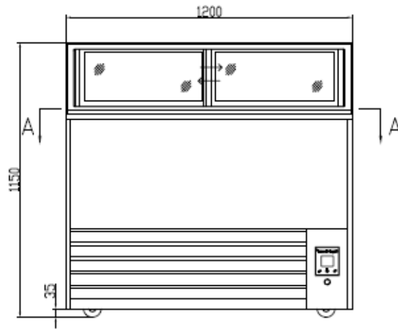
BACK 后视图
