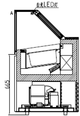
SECTION VIEW 左侧剖视图
