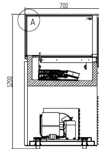
SECTION VIEW 左侧前视图
